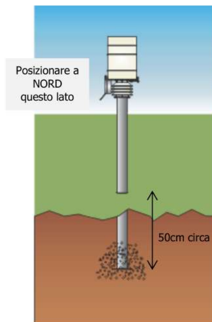
Versione con palo da 2m
